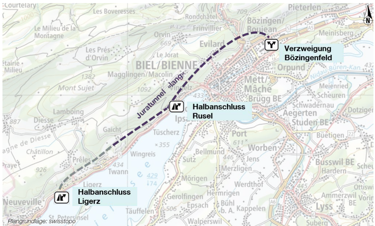
Abbildung 25 – Linienführung inkl. Verortung Anschlüsse vom MIV-Infrastrukturelement «Juratunnel lang»
